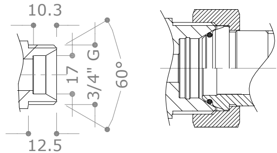
1007MS – Douille à souder \frac{3}{4} "F sf.x 15 mm
